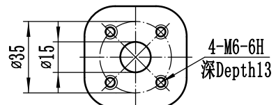
公制法兰油口 Metric split flange port
